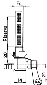
Figura 9 M 10x1 Conico 1:6
