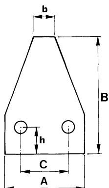
SEZIONE LAMA TIPO STRETTO (mm 51 - 2")
